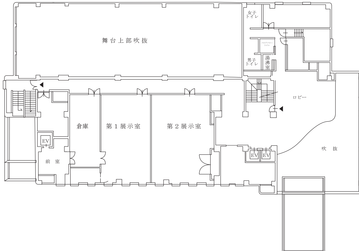
北館 2 F 平面図
