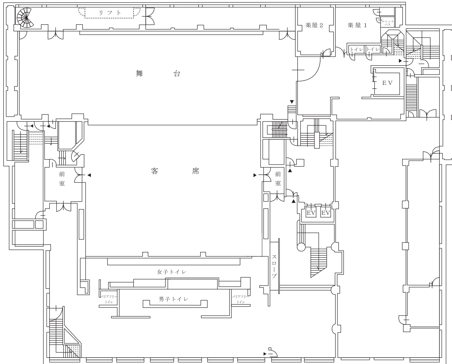
北館 B 3 F 平面図
