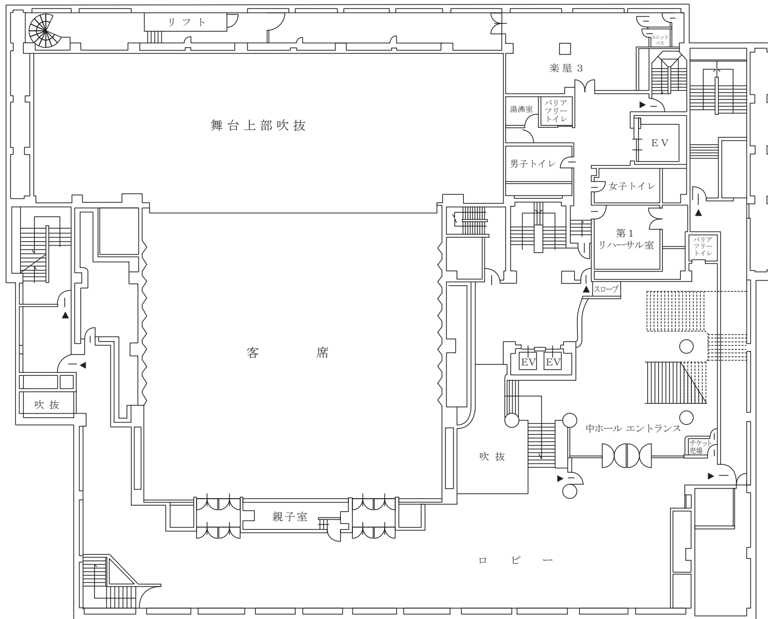
北館B 2 F 平面図
